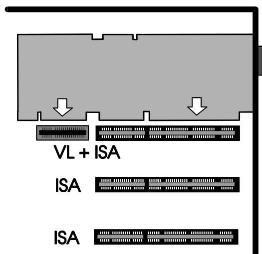
Instalación en una ranura de VESA Local Bus.
