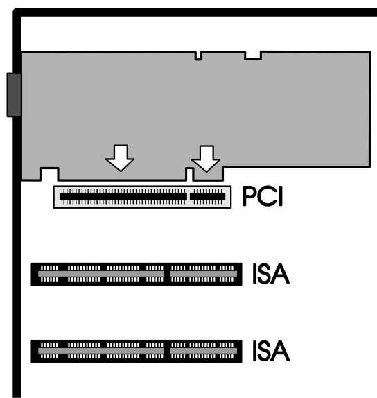
Instalación en una ranura de PCI.
