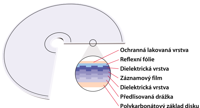
Skladba vrstev CD-RW média
