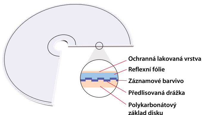
Řez médiem CD-R
