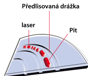
Záznamové pity jsou umístěny z pohledu čepce hlavy v prohlubni předlisované drážky (stopy)
